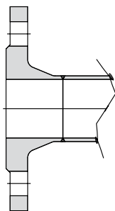
e.g. fixed flange acc. to DIN EN 1092-1 Type 11
